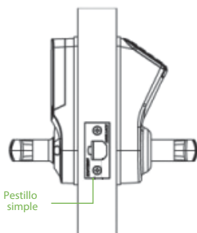
▲ Lado
