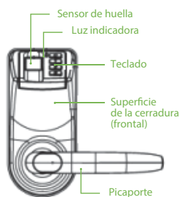
▲ Cerradura / frontal
